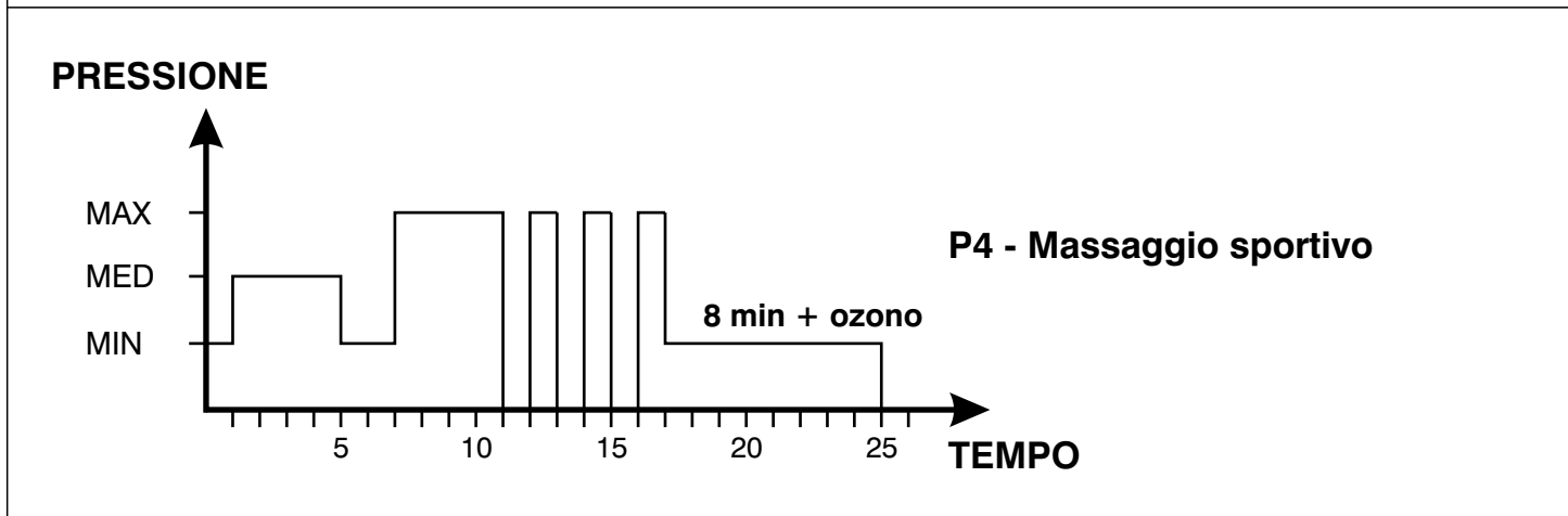
Diagrammi dell'andamento dei cicli di massaggio di ONDA e MAREA, macchine per idromassaggio con ozono.
